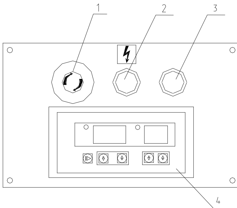
Рис.5. Расположение органов управления каландра гладильного ЛК1640
